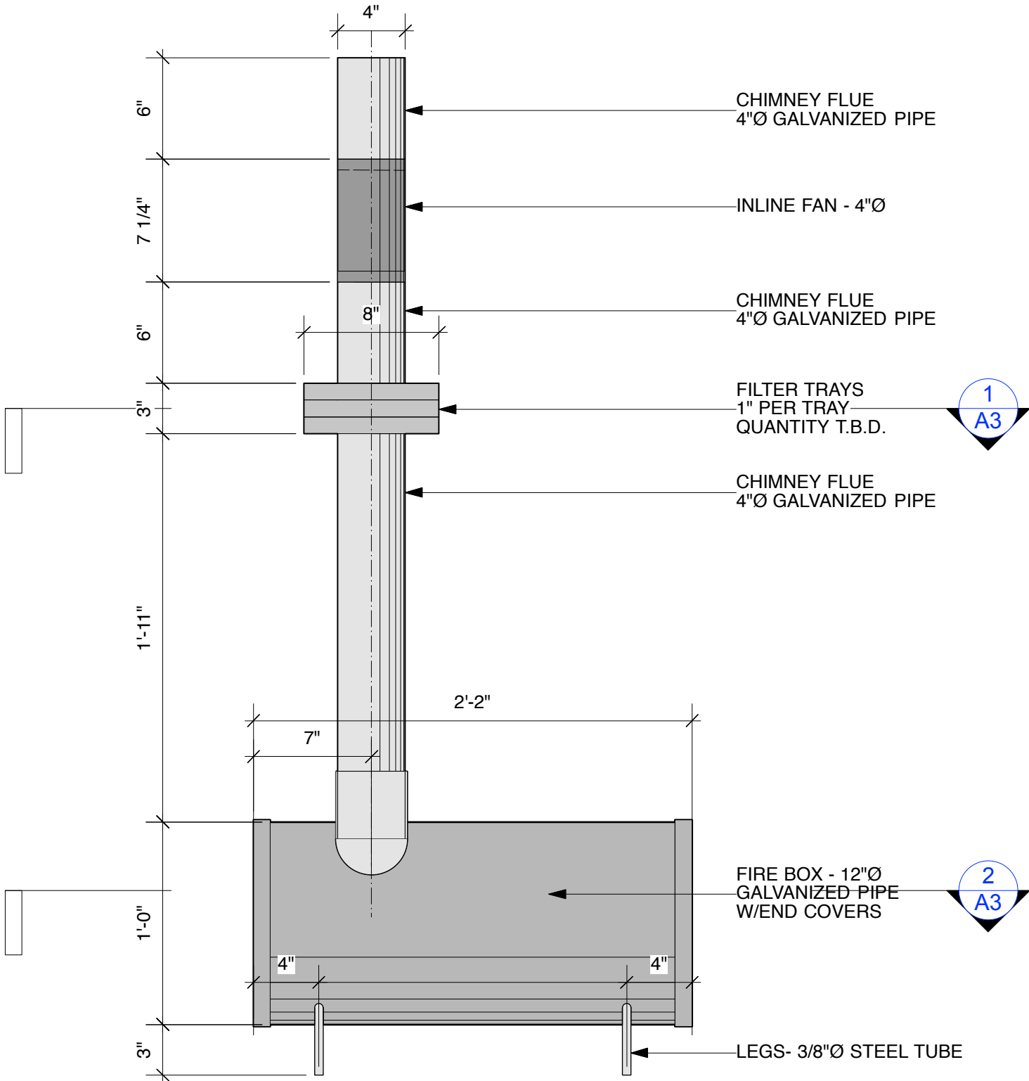
1 SIDE ELEVATION SCALE: 1 1/2"=1'-0"
